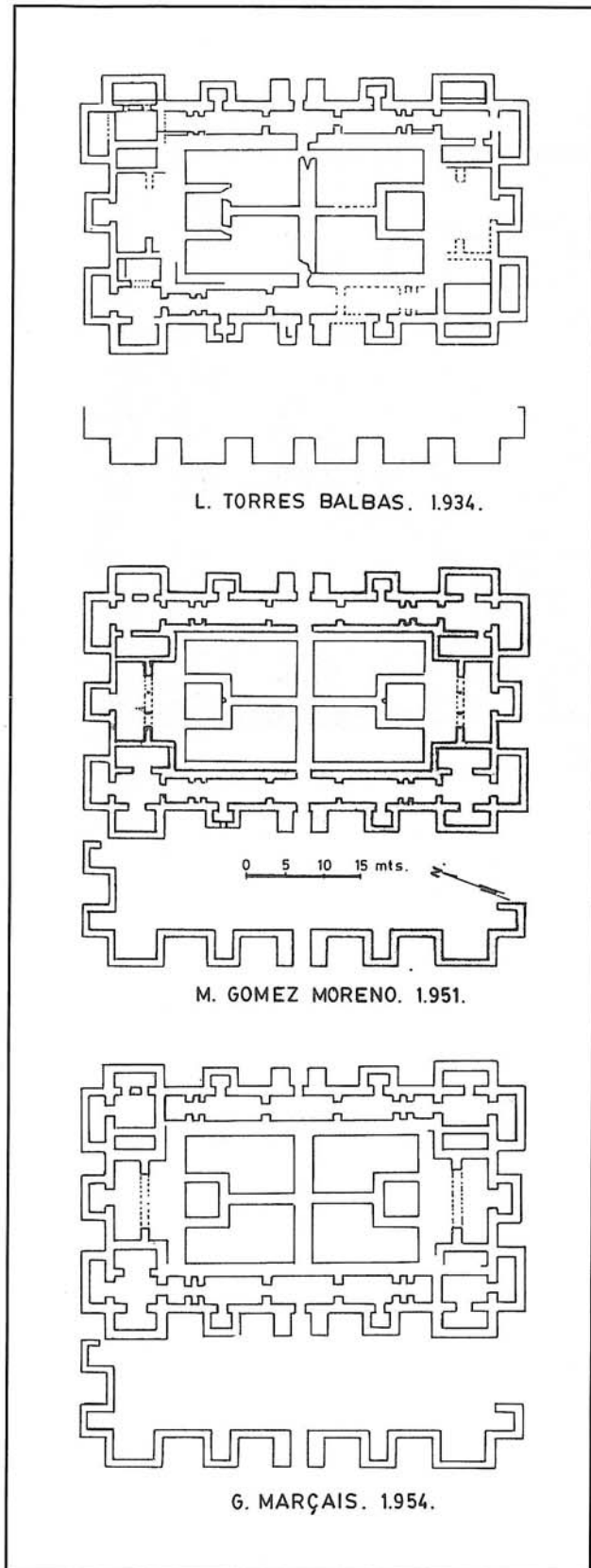
Fig. 6.- Plantas del Castillo de Monteagudo.
